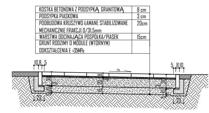
PRZEKRÓJ A-A 1:50
